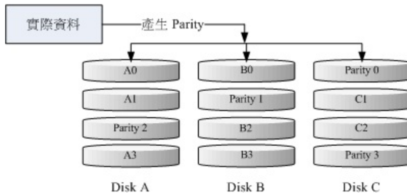
图14.2.4、RAID-5 的磁盘写入示意图
