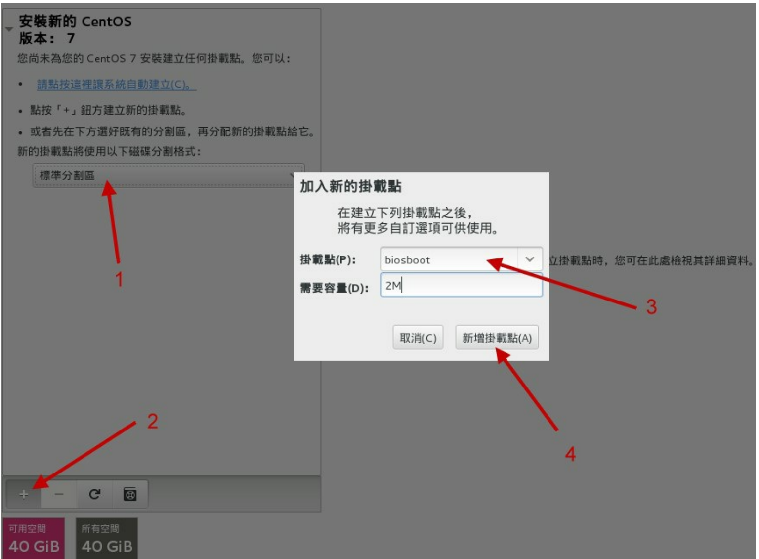
图3.2.21、创建 BIOS boot 分区的示意图
