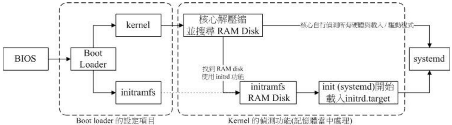
图19.1.3、BIOS 与 boot loader 及核心载入流程示意图
