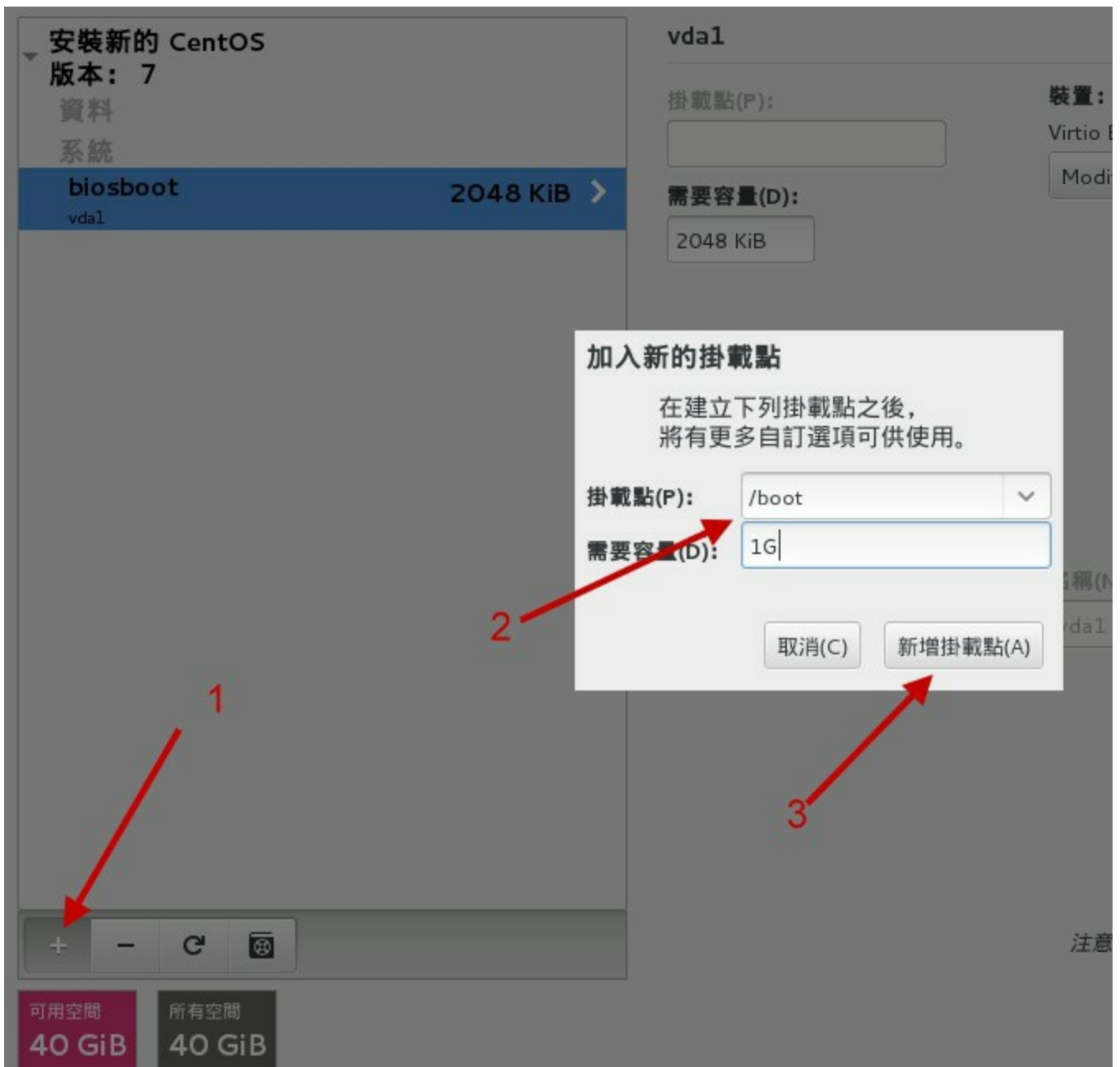
图3.2.23、创建 /boot 分区的示意图
